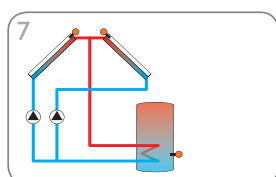
Zonne-energiesysteem met oost-/westdak (pagina 14)
