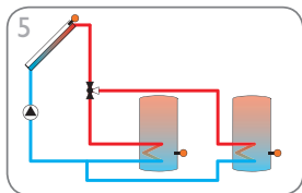
Zonne-energiesysteem met 2 boilers en kleplogica (pagina 12)
