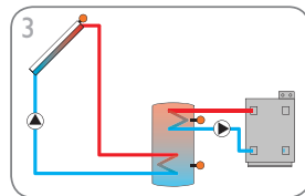
Zonne-energiesysteem met 1 boiler en naverwarming (pagina 10)
