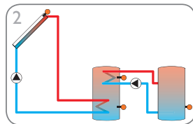
Zonne-energiesysteem met 2 boilers en warmte-uitwisseling (pagina 9)
