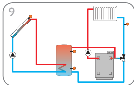
Zonne-energiesysteem met 1 boiler en retourverhoging (pagina 16)
