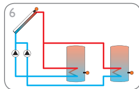
Zonne-energiesysteem met 2 boilers en pomplogica (pagina 13)
