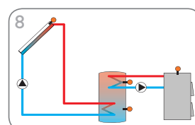
Zonne-energiesysteem met 1 boiler en vaste brandstofketel (pagina 16)
